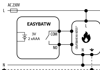
в) Схема на свързване към клемна шина
